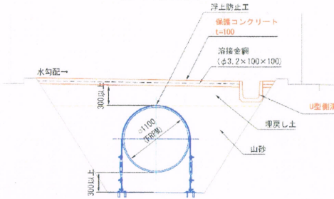
標準断面図
